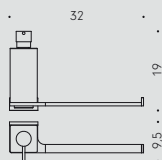
B1674 Spandisapone (L 0,31) e porta salvietta per bidet destro Right soap dispenser and towel holder for bidet
