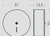
B9983N Distributore per rotoli di carta igienica con serratura di sicurezza - acciaio inox. Dimensioni max rotolo inseribile: diametro 300mm Stainless steel toilet roll dispenser with safety lock. Maximum dimensions of inserted roll: 300 mm diameter
