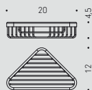
B2732 Basic Angolare semplice Single corner basket
