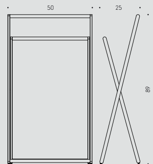
B9737 Cavalletto porta salviette H.89 Rack
